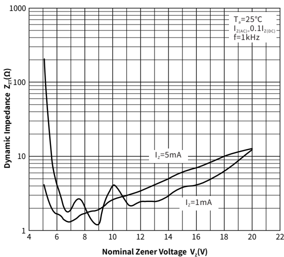
Fig. 5 Effect of Zener Voltage on Zener Impedance
